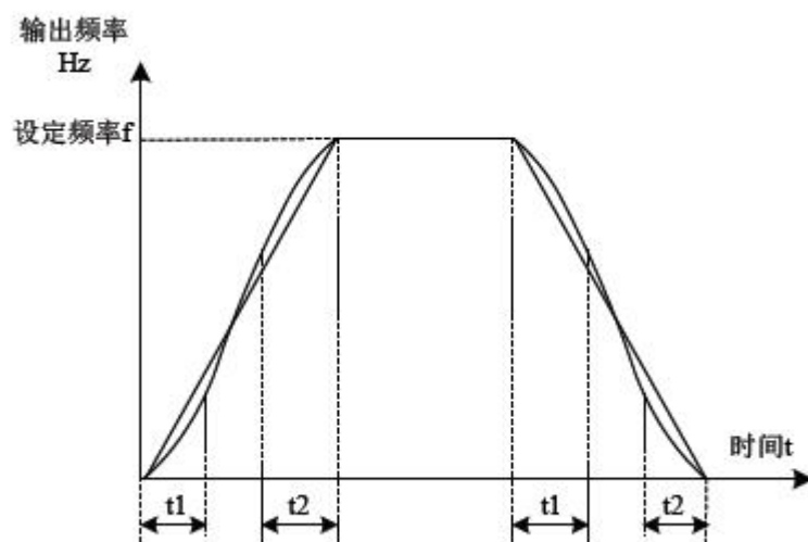
图 10 变频器的频率特性 (频率上升时间、频率下降时间)
