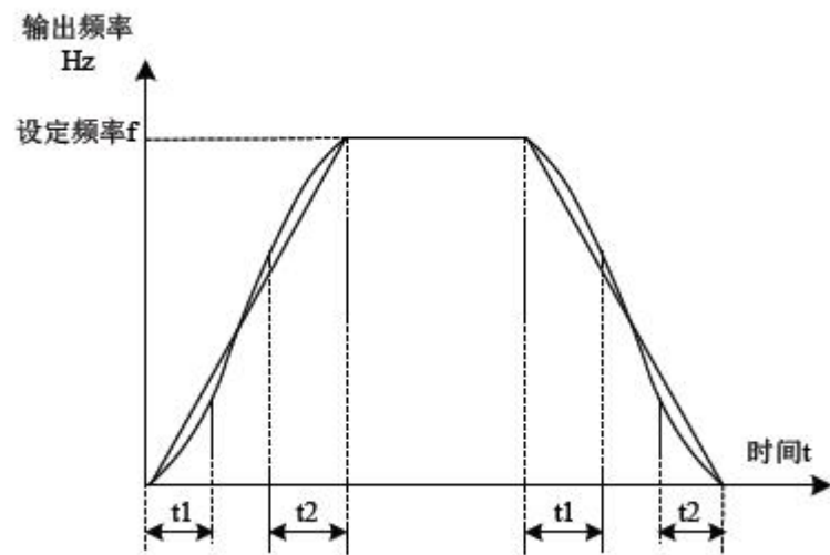
图 7-1 变频器的频率特性 (a) 恒转矩变频特性 (b) 恒功率变频特性
